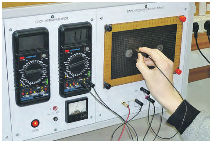
Лабораторная работа по исследованию электростатического поля
